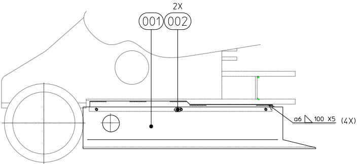
Zijaanzicht
